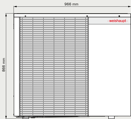
Außengerät WSB 6 – 10
