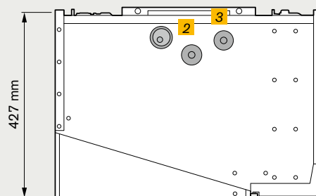
Geräteunterseite
