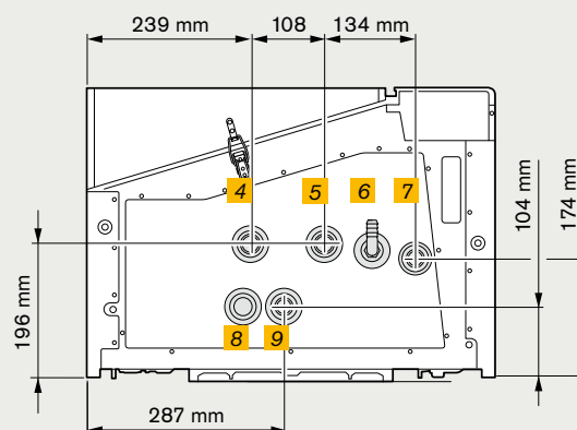
Geräteunterseite
