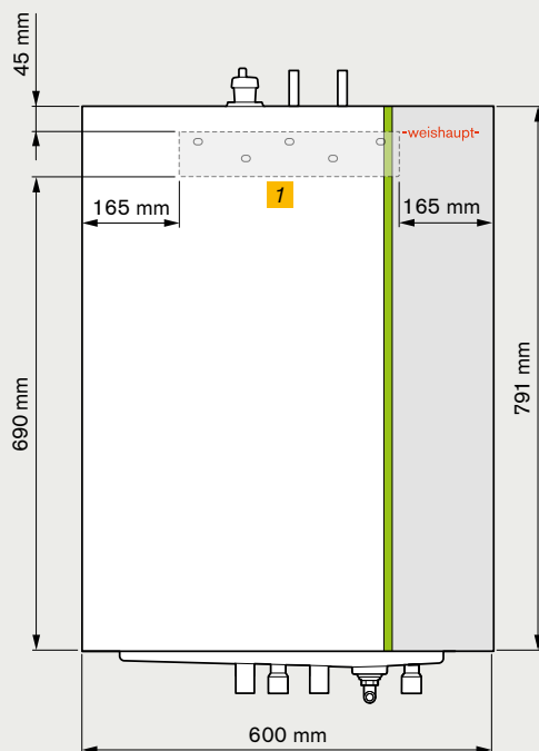
Gerätefront
